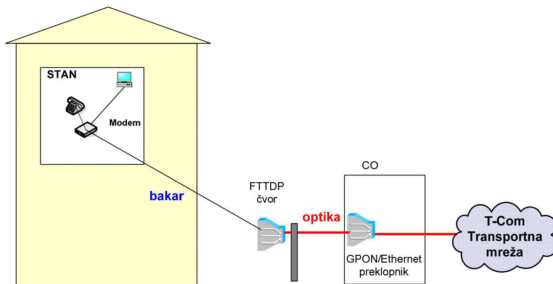
Slika 35. Način realizacije FTTDP koncepta u pristupnoj mreži
