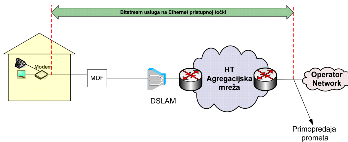
Slika 14. Veleprodajni širokopolasni pristup za pružanje VoIP usluge na Ethernet razini u slučaju kada krajnji korisnik ostvaruje Osnovni pristup mreži putem usluge HT-a
